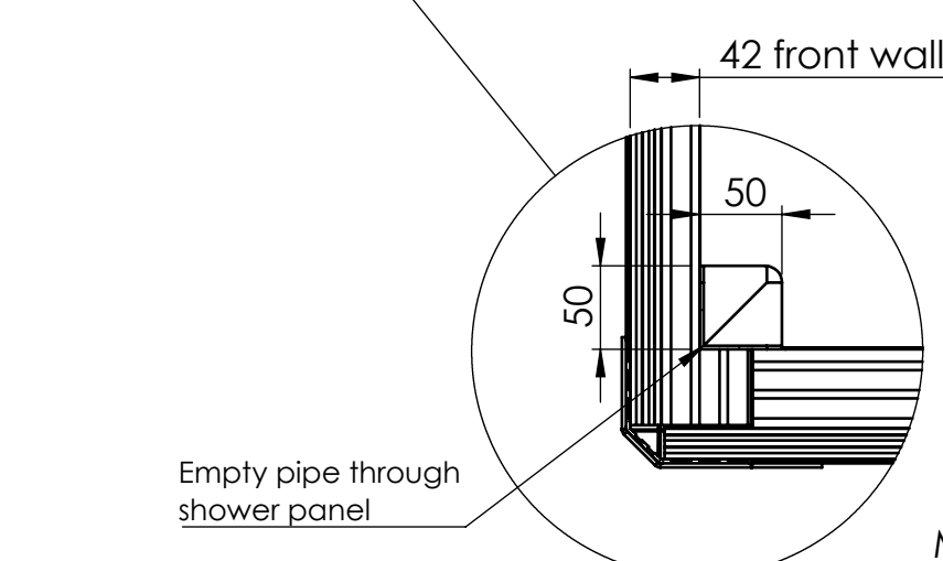
DETAIL GD MAßSTAB 1 : 5
